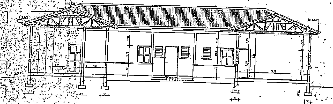
COUPE TRANSVERSALE SUR AILES
