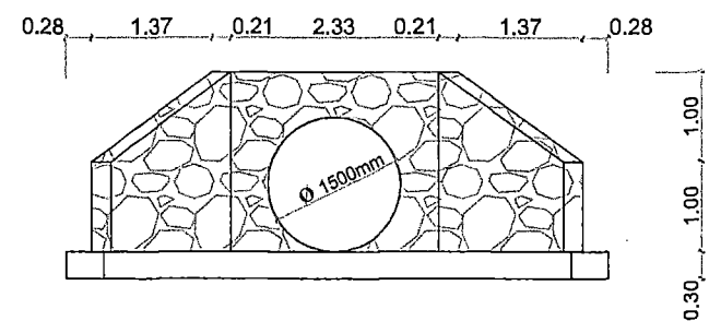
RIGHT ELEVATION
