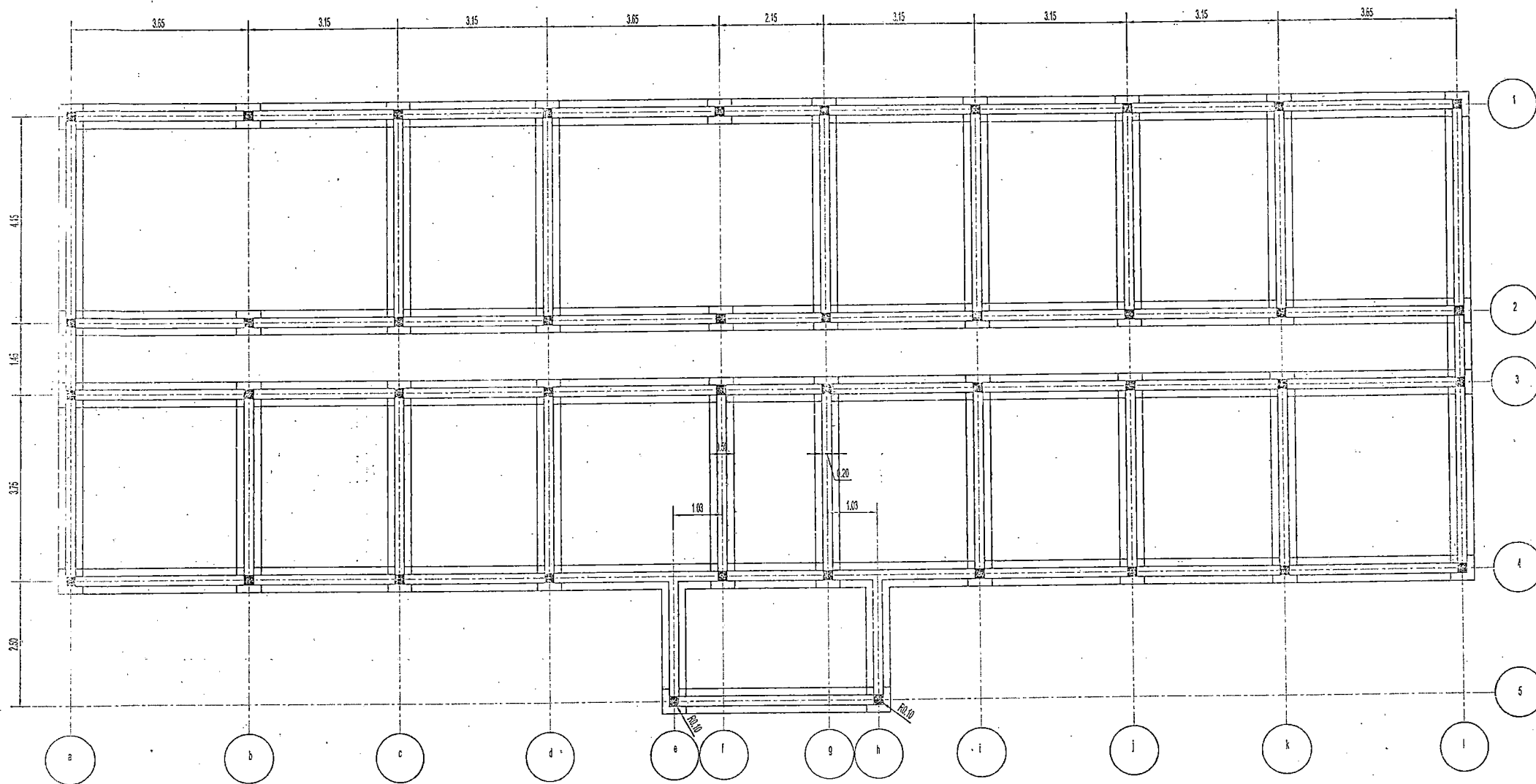
PLAN DE FONDATIONS
