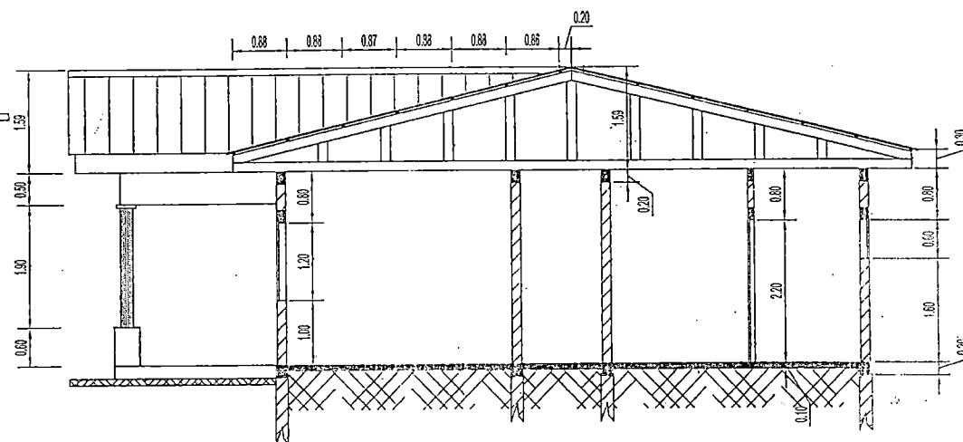
COUPE A-A
