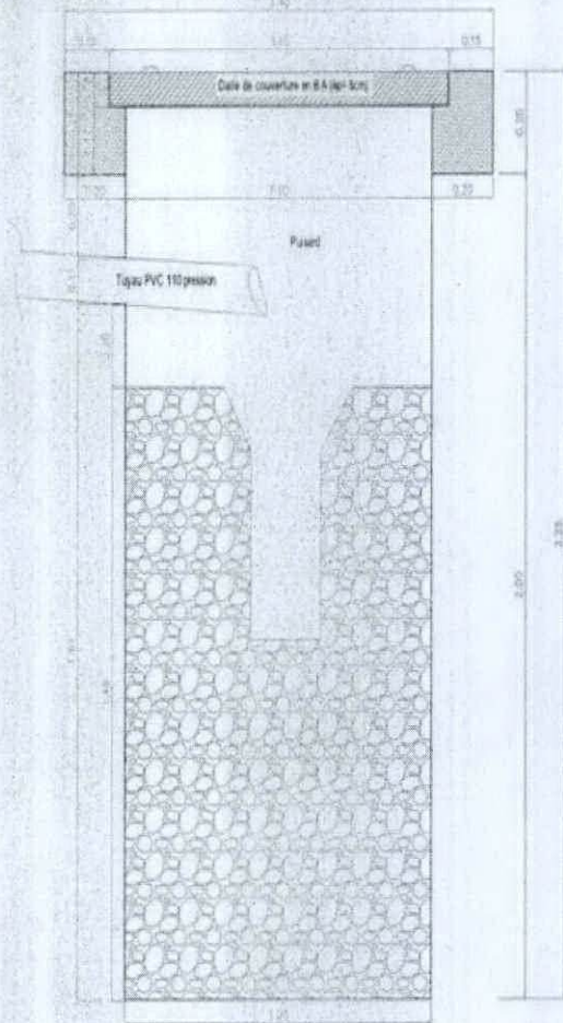
COUPE B-B
