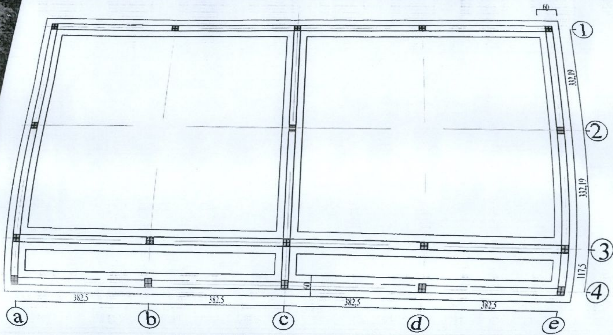
PLAN DE FONDATIONS
