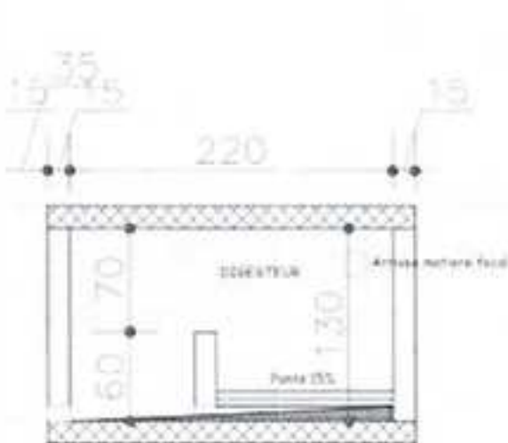
COUPE CC - SECTION CC
