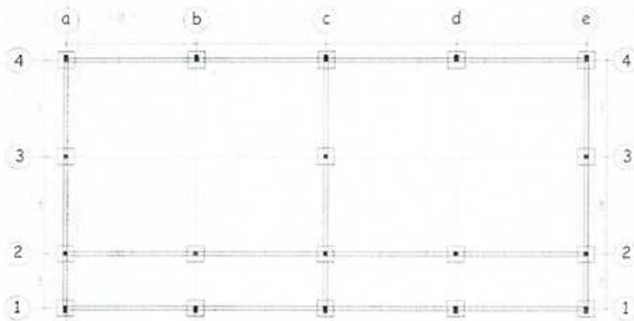
PLAN DE FONDATION - FOUNDATION PLAN
