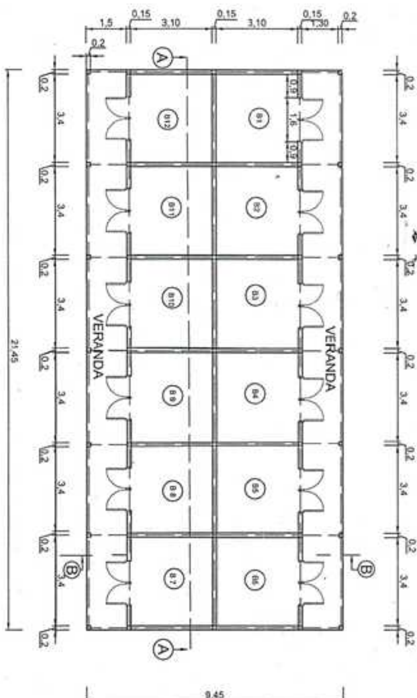
TRAVAUX DE CONSTRUCTION DES 12 BOUTIQUES AU CENTRE COMMERCIAL DE TIBATI PLAN DE DISTRIBUTION ECHELLE: 1/1
