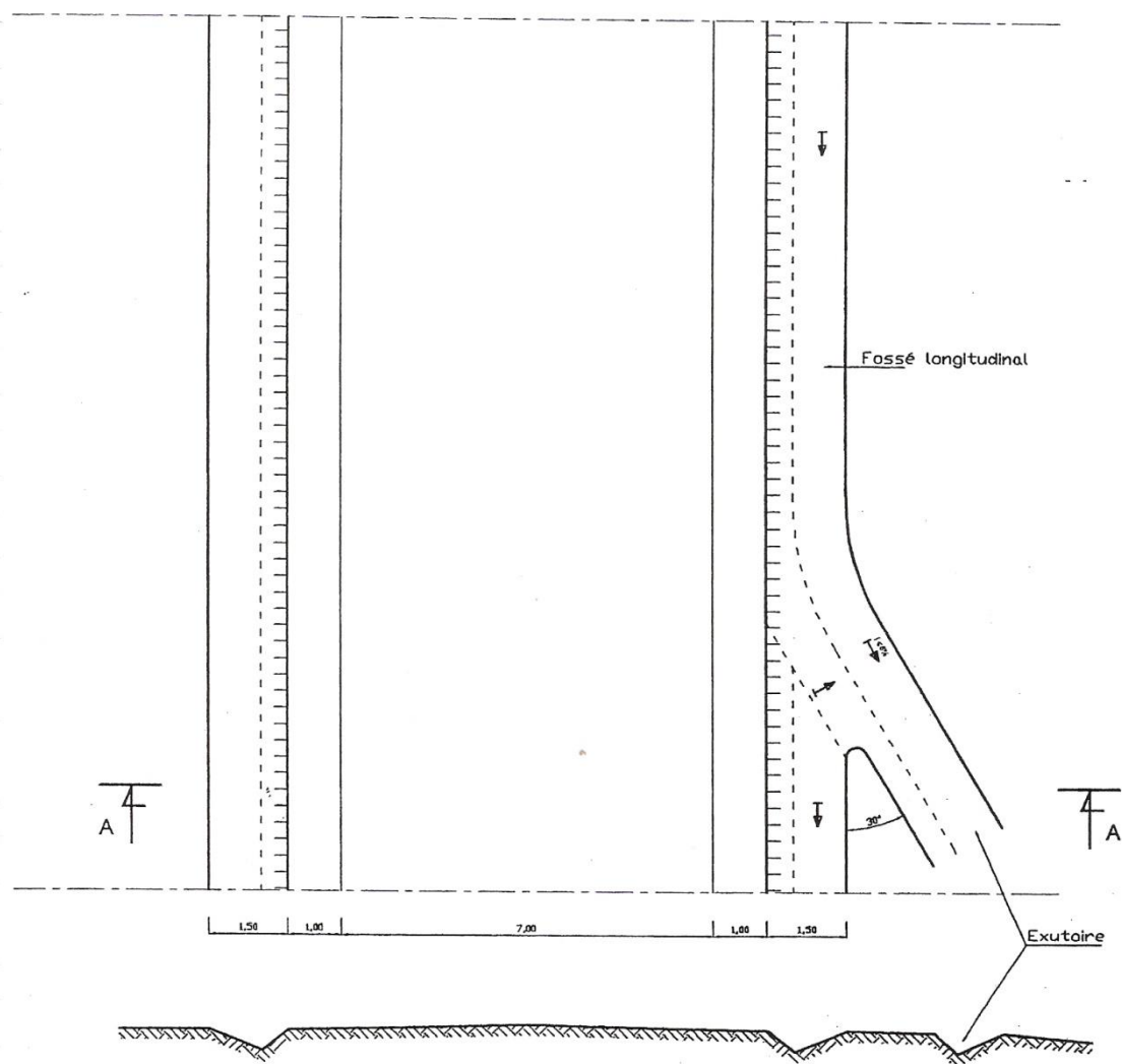
COUPE A-A
