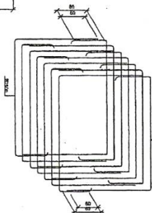
CADRES EXTÉRIEURS PROFILS ALUMINIUM
