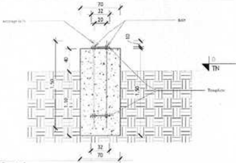
2 Coupe 1 1:25
