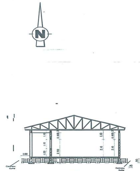
COUPE A-A SECTION A-A
