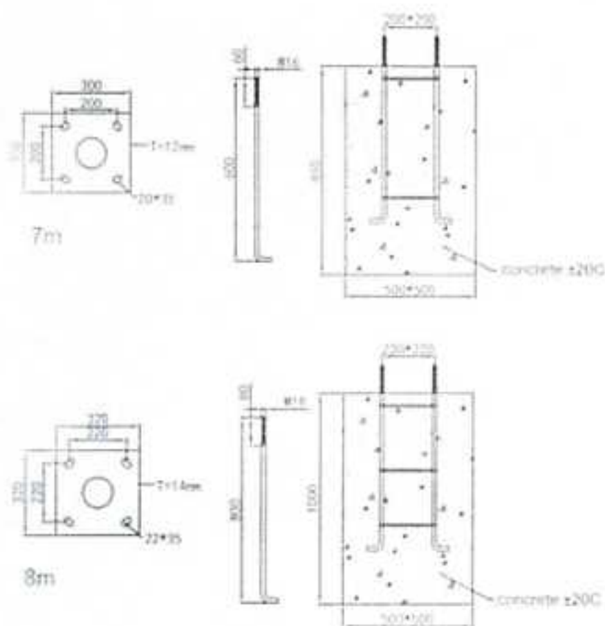
boulons d'ancrage et taille de la base en béton pour le lampadaire
