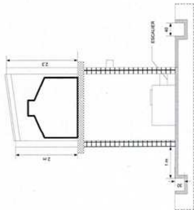
COUPE AA
