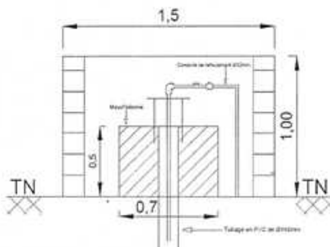
AMENAGEMENT DE LA TETE DU FORAGE
