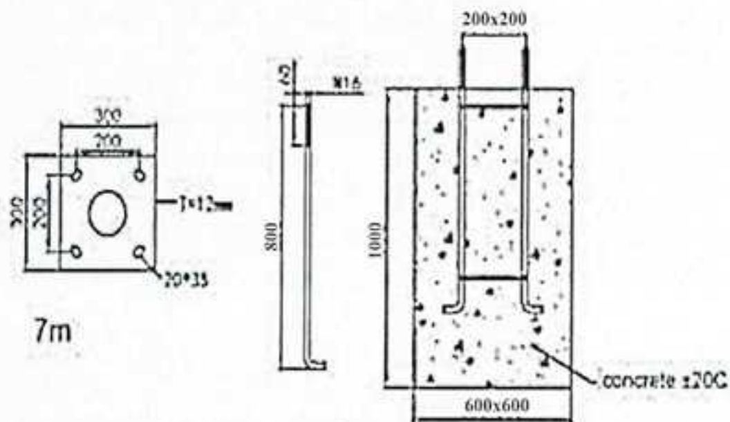
Boulons d'ancrage et taille de la base en béton pour le lampadaire
