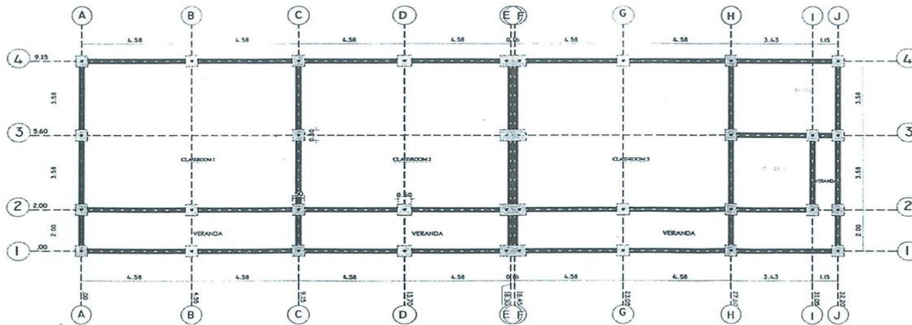
PLAN DE FONDATION FOUNDATION PLAN
